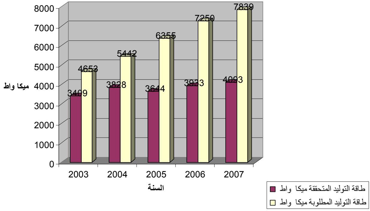
شكل رقم (1) طاقة التوليد المتحققة والمطلوبة للسنوات 2003-2007 (ميكا واط)
